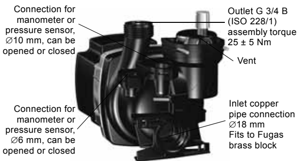
CESAO2 composite end-suction air outlet
