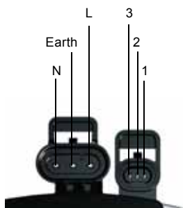
Fig. 63 Connections Mini SS
