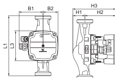
Dimensions
