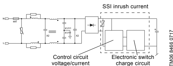
Fig. 60 SSI
