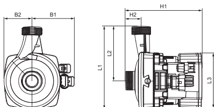
Dimensions
