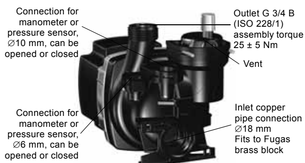
CESAO2 composite end-suction air outlet
