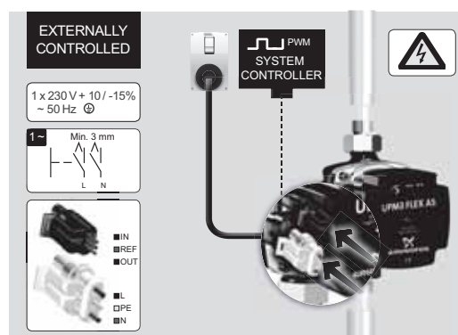
Fig. 65 Control box with Mini SS connection
